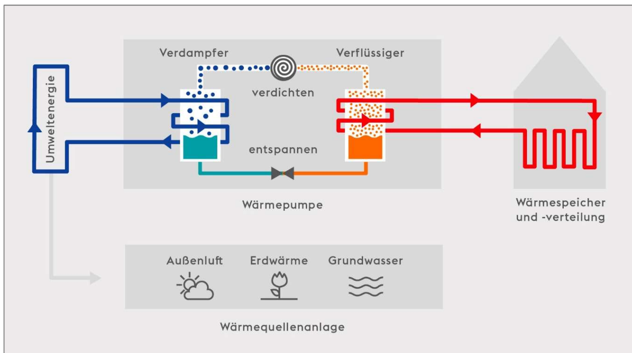
Abbildung 22: Prinzipschema Luft-Wärmepumpe (Grafik: proKlima - Der enercity-Fonds)
