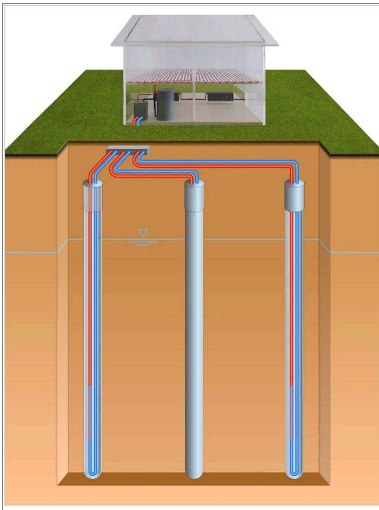
Abbildung 25: Gebäude mit Erdwärmesonden (Grafik: Landesamt für Bergbau, Energie und Geologie)
