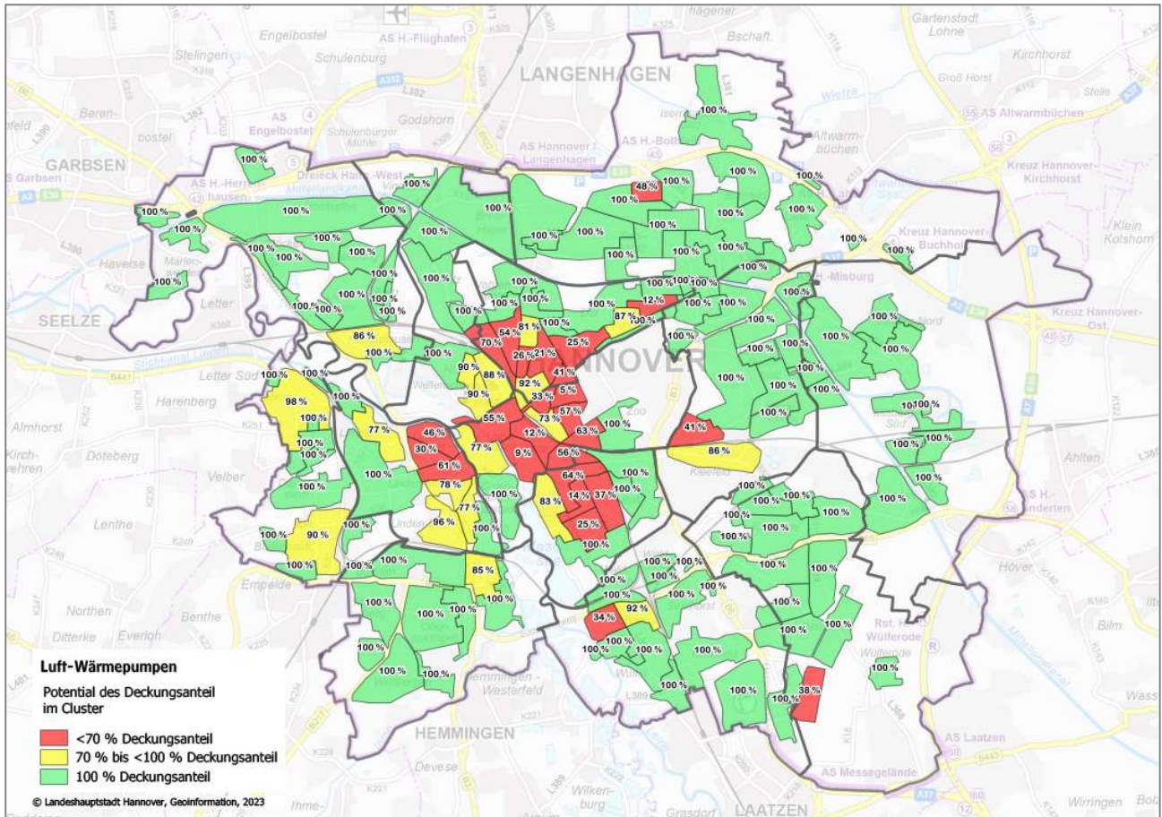
Abbildung 23: Potenzialkarte Luft-Wärmepumpen
